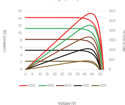
Curvas de corriente-voltaje y potencia-voltaje (590W)
